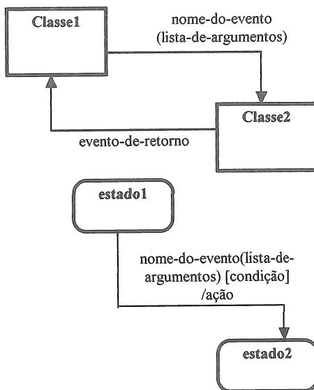
Notação OMT
